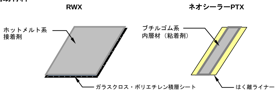
図 1 構 造
